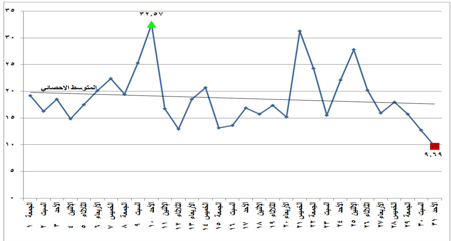
شكل (٢٥) الطاقة الكهربائية المنتجة من الرياح والشمس خلال شهر يناير ٢٠٢١
