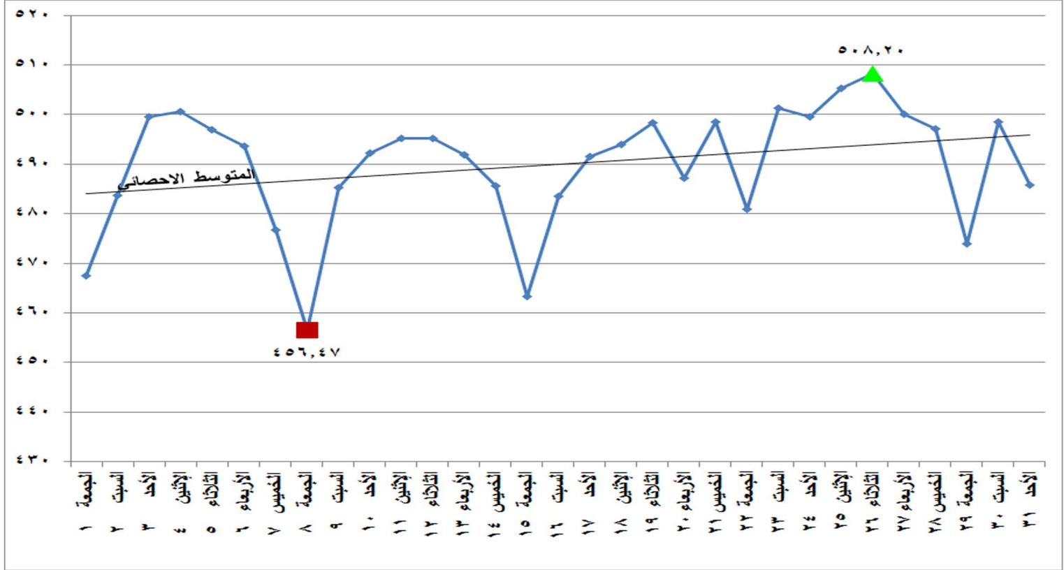
شكل (١٥) إجمالي الطاقة الكهربائية المنتجة من كل المصادر الأولية خلال شهر يناير ٢٠٢١
