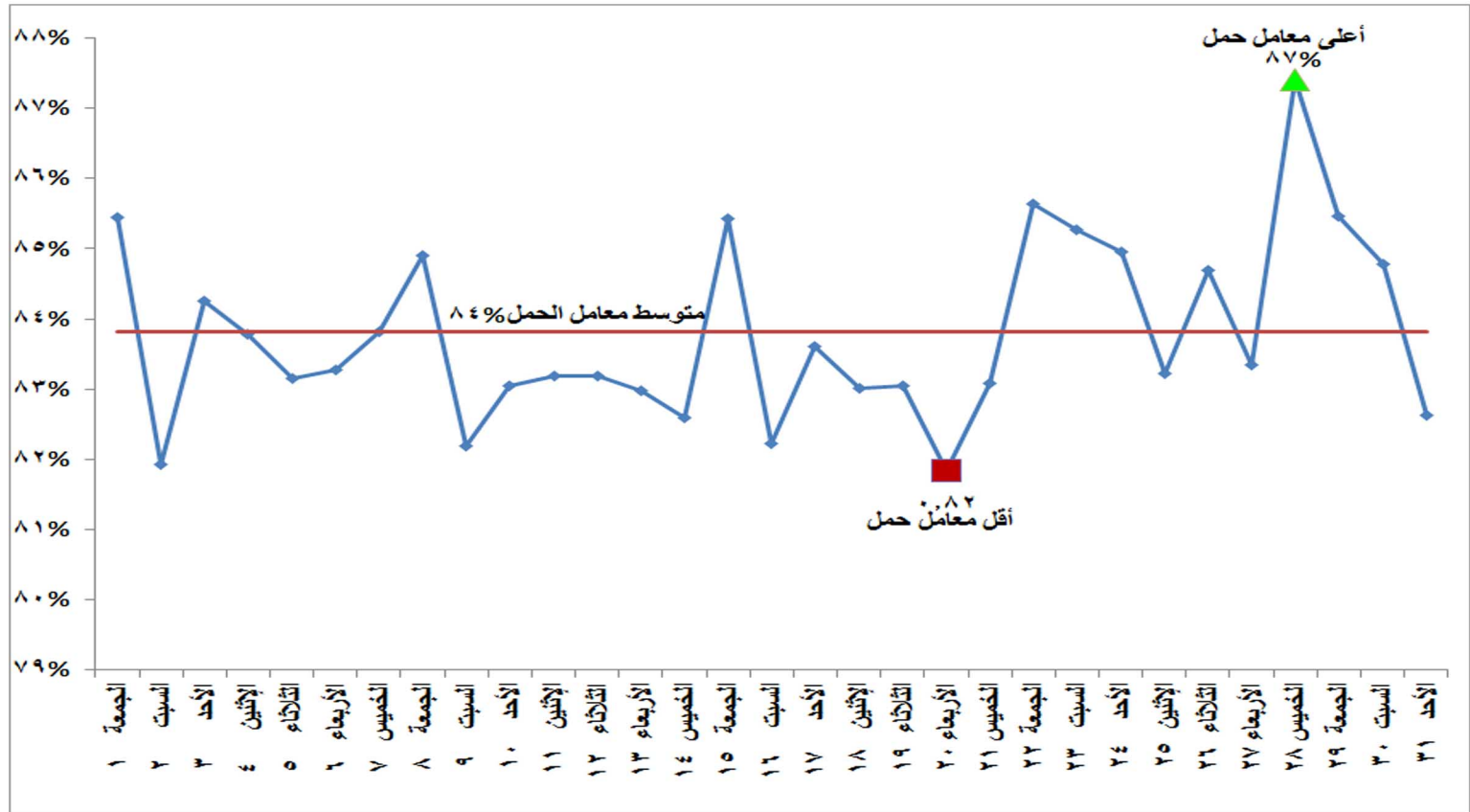
شكل (١٢) إجمالي معامل الحمل لوحدات الانتاج خلال شهر يناير ٢٠٢١
