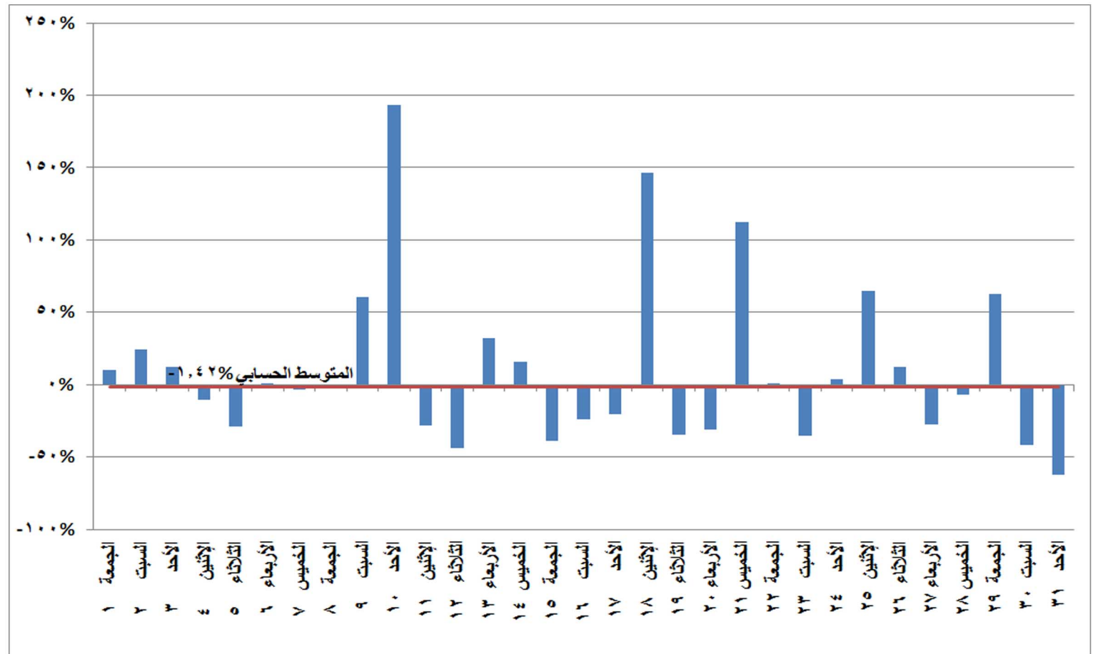
شكل (٢٦) نسب التغير في استخدام الرياح والشمس في إنتاج الطاقة الكهربائية خلال شهر يناير ٢٠٢١ مقارنة بالشهر المماثل من العام السابق
