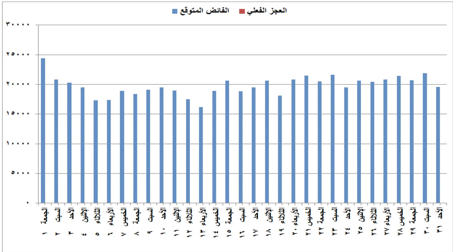
شكل (٧) الفااض والعجز المتوقع للقدرات خلال شهر يناير ٢٠٢١
