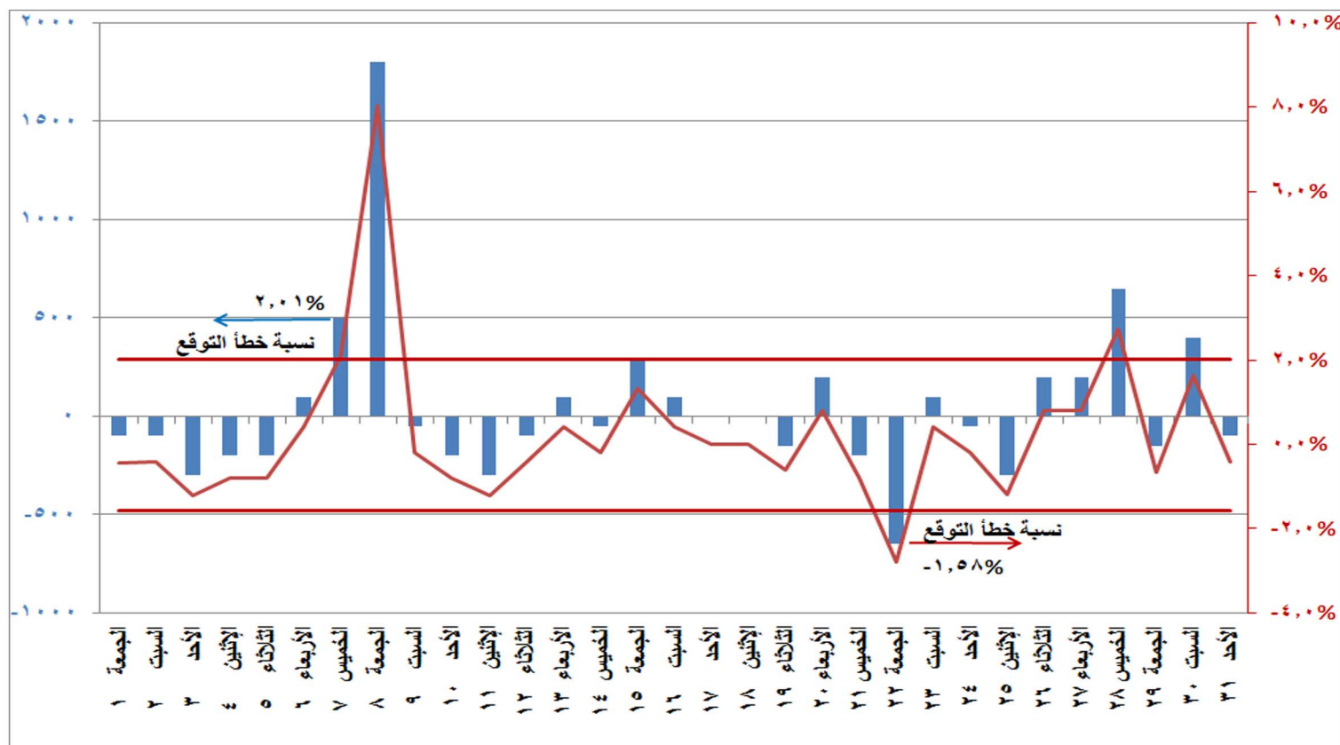
شكل (١٠) الفرق بين الحمل الأقصى المتوقع والمسجل فعليا ونسبة الفرق إلى الحمل المسجل فعليا خلال شهر يناير ٢٠٢١
