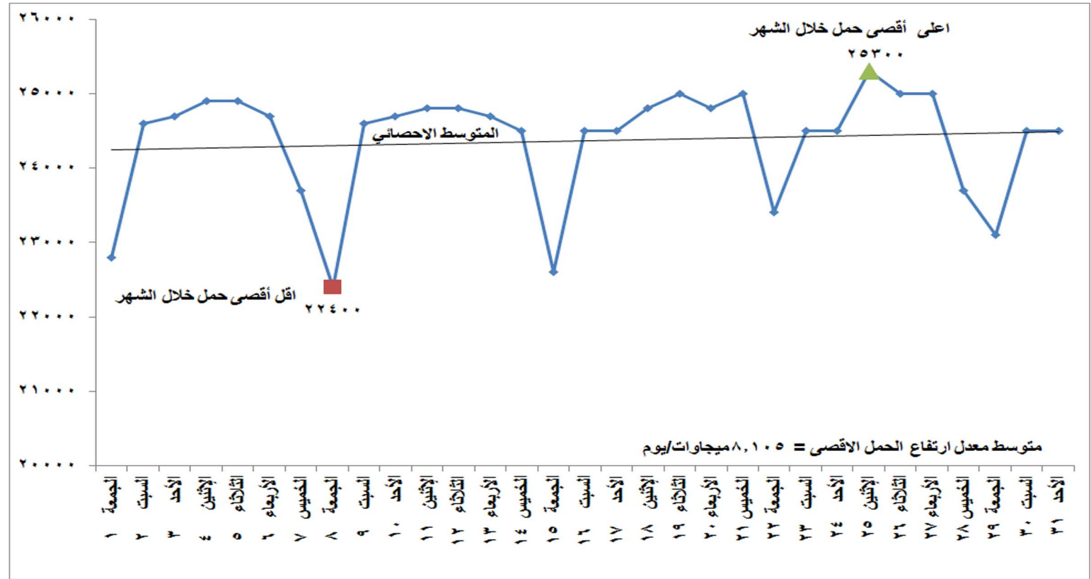
شكل (١) تطور الحمل الأقصى اليومي خلال شهر يناير ٢٠٢١
