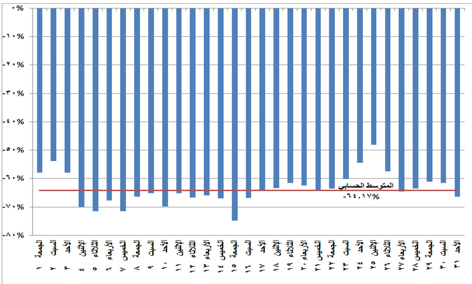
شكل (٢٠) نسب التغير في استخدام المازوت في إنتاج الطاقة الكهربائية خلال شهر يناير ٢٠٢١ مقارنة بالشهر المماثل من العام السابق
