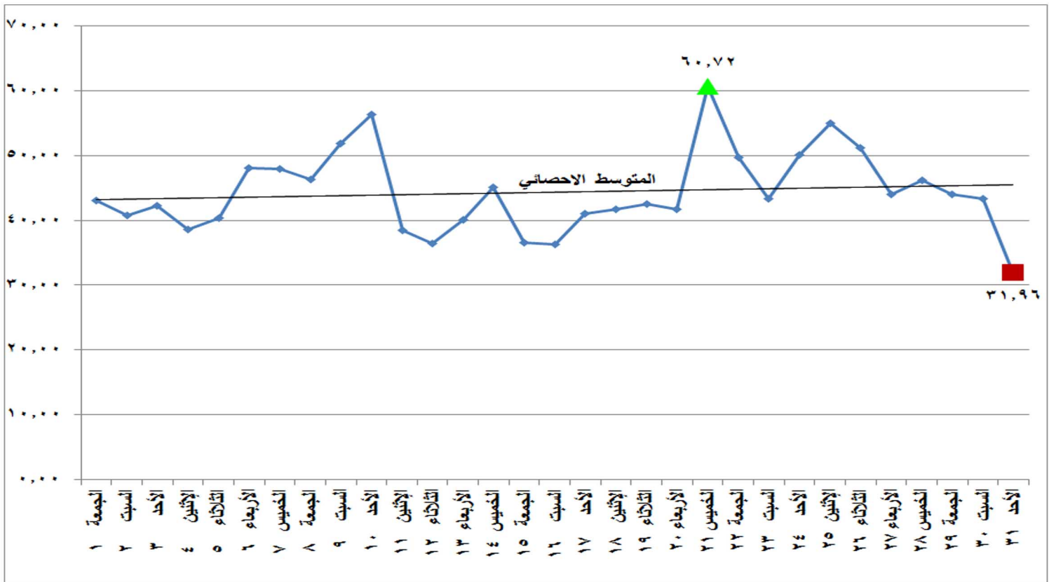
شكل (٢١) الطاقة الكهربائية المنتجة من المصادر غير الحرارية خلال شهر يناير ٢٠٢١
