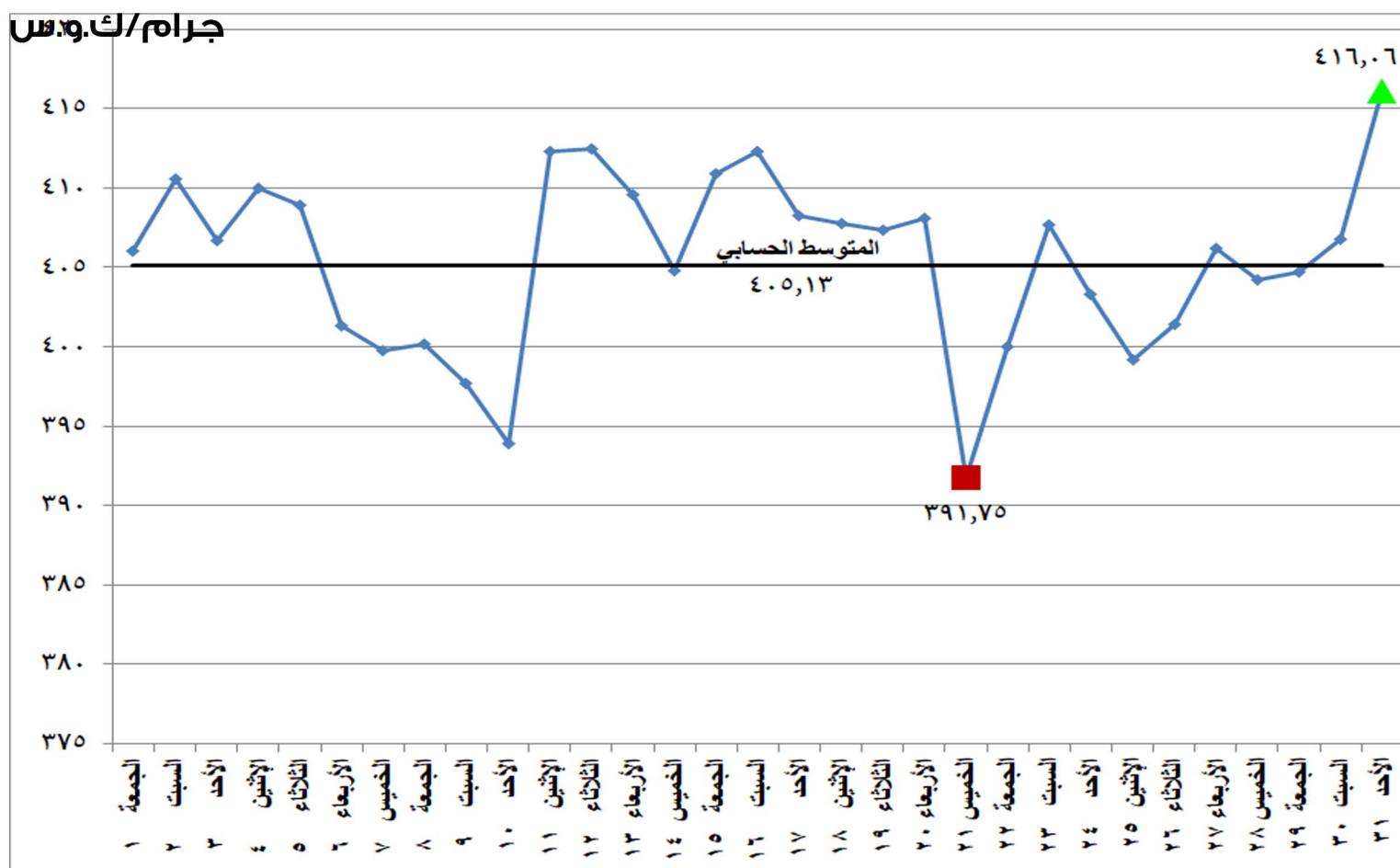
شكل (١٤) معامل انبعاثات غاز ثاني اكسيد الكربون المكافئ على مدى شهر يناير ٢٠٢١
