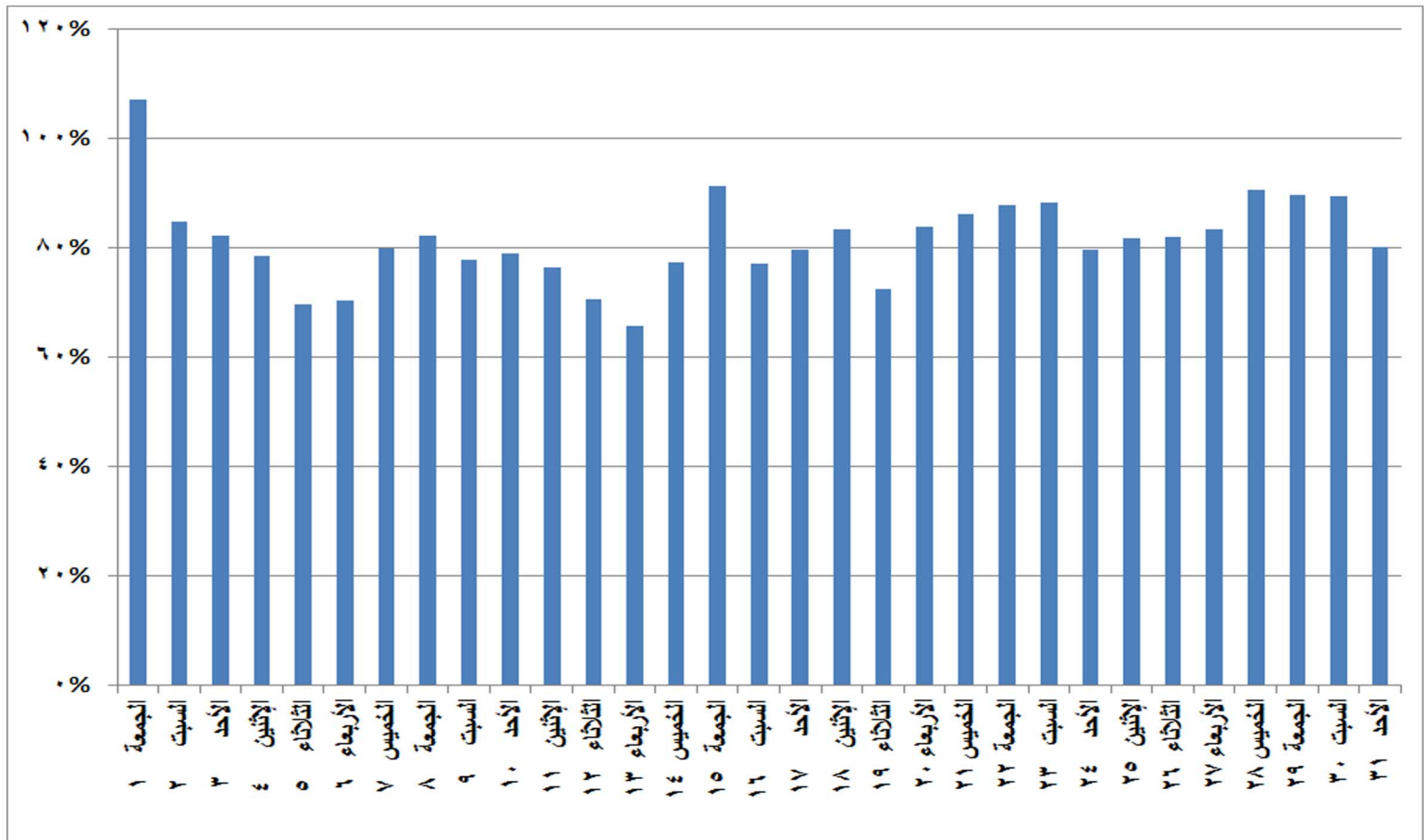
شكل (٢٨) نسب الفائض للحمل الاقصى المسجل يوميا خلال شهر يناير ٢٠٢١
