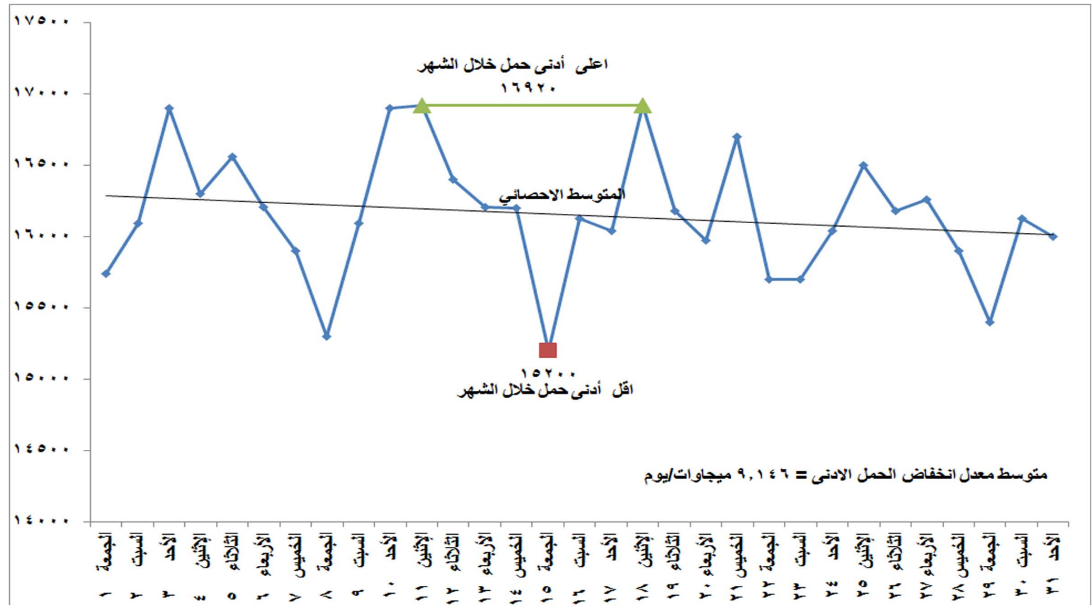
شكل (٢) تطور الحمل الأدنى اليومي خلال شهر يناير ٢٠٢١
